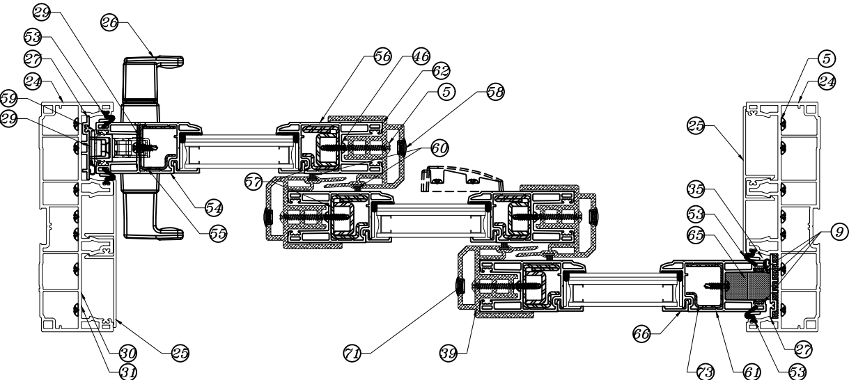
SECTION D-D
