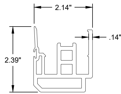
INTERLOCK 6063-T5 ALUMINUM
